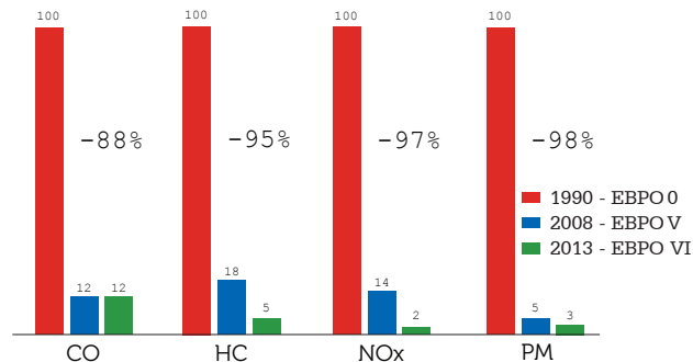
Сокращение выброса вредных веществ тяжелыми коммерческими автомобилями
